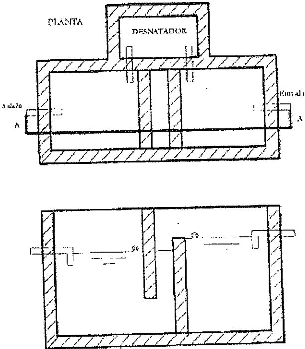
Ilustración No. 1 –Detalle del diseño de la Trampa de Grasas hermética construida en la EDS SANTA ANA –BARANOA.
