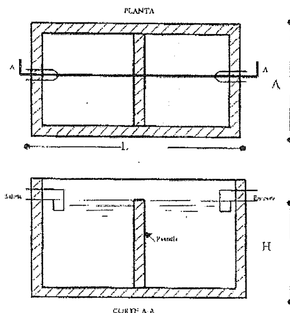
Figura 1. Sedimentario primario.
